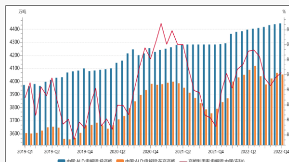
图5 近年中国电解铝产能及产能利用率情况
