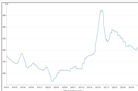
图4 近年国内氧化铝价格走势
