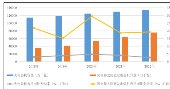
图2 近年中国发电装机容量变动情况
