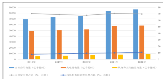
图3 中国发电量、用电量情况
