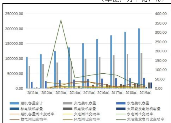
图4 近年中国发电装机容量变动情况 (单位：万千瓦、%)
