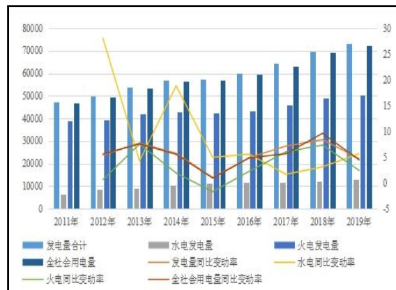
图5 中国发电量、用电量及增幅情况
