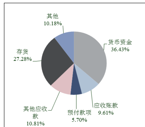
图6 公司2019年底流动资产构成情况
