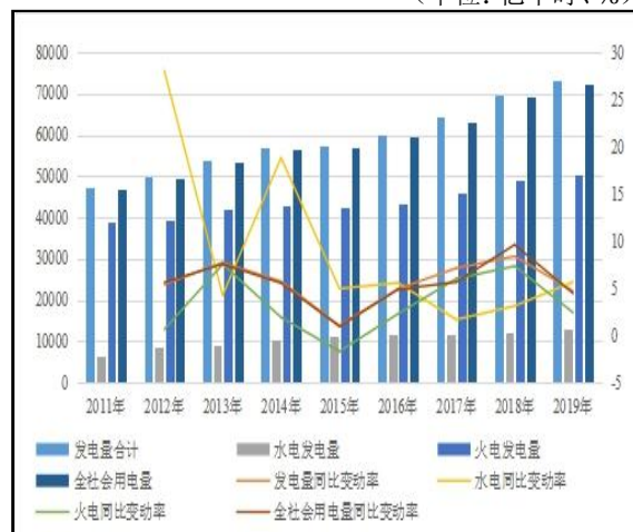
图5 中国发电量、用电量及增幅情况 (单位:亿千瓦时、%)
