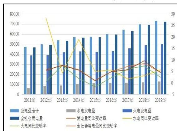
图5 中国发电量、用电量及增幅情况 (单位:亿千瓦时、%)
