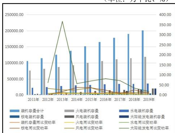
图4 近年中国发电装机容量变动情况 (单位:万千瓦、%)
