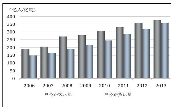
图3 2006-2013年全国公路运输量情况
