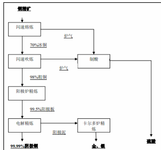
图 7 公司生产工艺流程图
