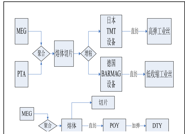
图 4 公司产品生产工艺及流程
