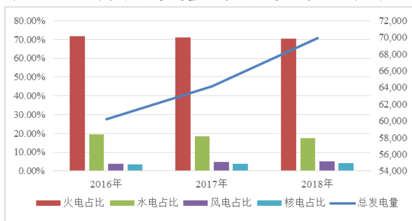
图2 2016~2018年中国电力发电总量以及来源占比情况（单位：亿千瓦时，%）
