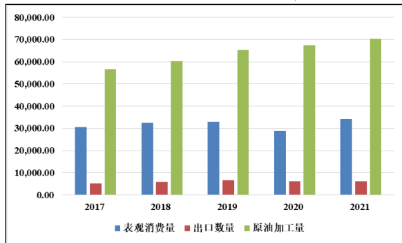
图 4 2017 年以来成品油生产及出口情况
