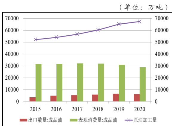
图 4 2015 年以来成品油生产及出口情况
