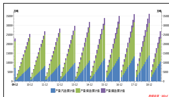
图4 成品油产量情况（单位：万吨）
