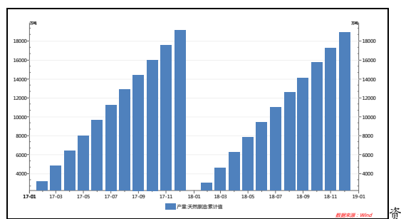
图 1 近年来中国原油产量情况
