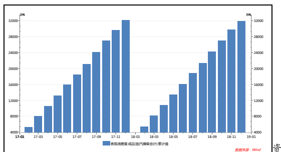
图 3 成品油消费量情况
