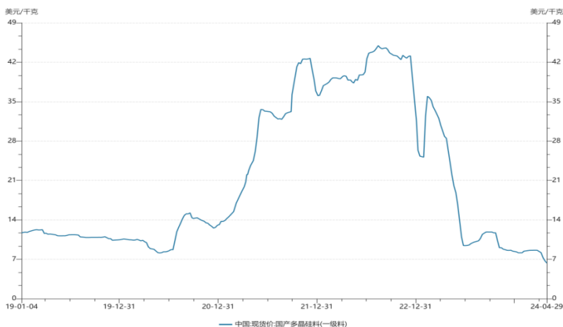
图表 1 • 2019 年以来光伏级多晶硅现货价
