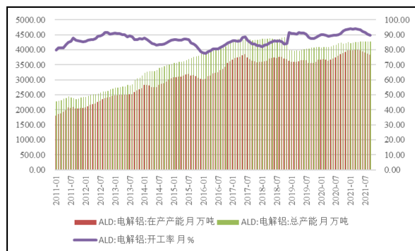
图4 近年中国电解铝产能及产能利用率情况 (单位：万吨/年、%)
