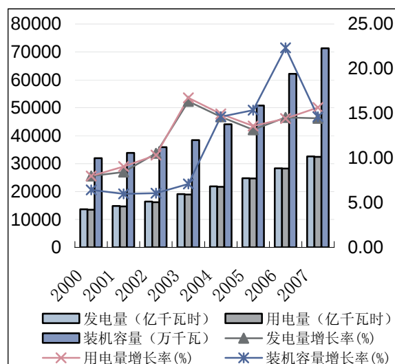
图1 近年中国电力供求状况
