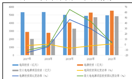
图1 近年中国电源及电网投资情况
