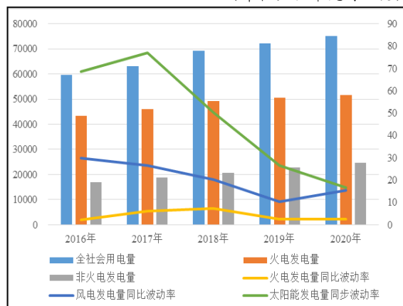
图3 中国发电量、用电量及增幅情况 (单位: 亿千瓦时、%)
