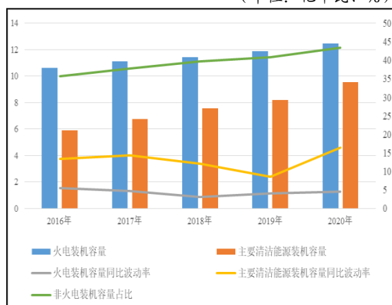
图2 近年中国发电装机容量变动情况 (单位: 亿千瓦、%)
