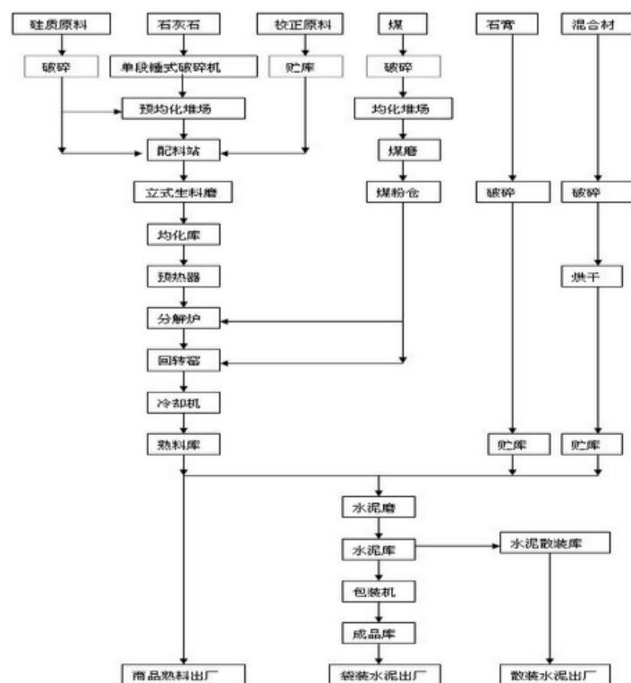
图7 公司水泥生产工艺图
