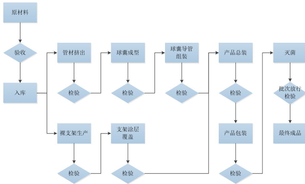
图 7 心脏支架工艺流程图
