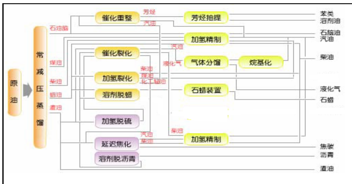
图3 炼油工艺流程图
