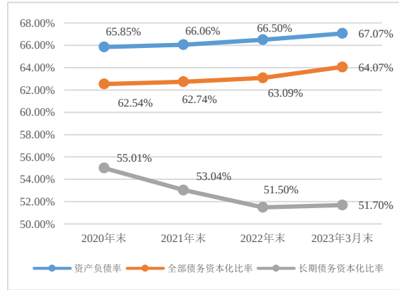
图 3 2020 - 2022 年末及 2023 年 3 月末公司债务杠杆水平
