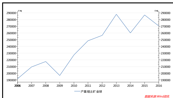
图1 全球铝土矿产量情况
