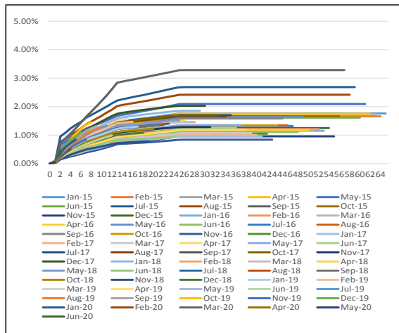
图2 静态池在后续月份的30天以上累计逾期率表现
