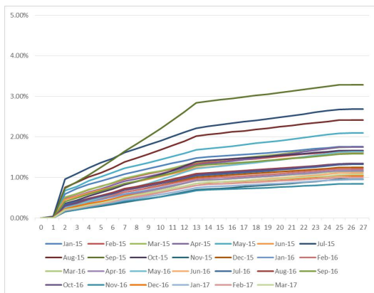
图 2 静态池在后续月份的 30 天以上累计逾期率表现图
