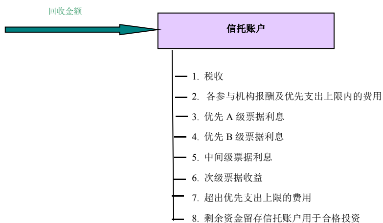
附图 1-1 循环期内现金流分配
