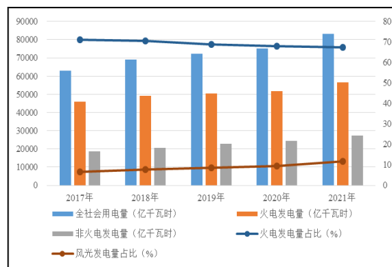
图3 中国发电量、用电量情况
