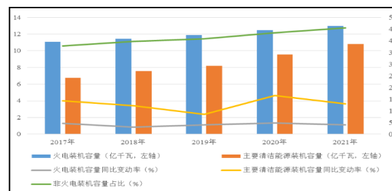
图2 近年中国发电装机容量变动情况
