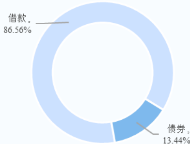
公司 2025 年末债务构成
