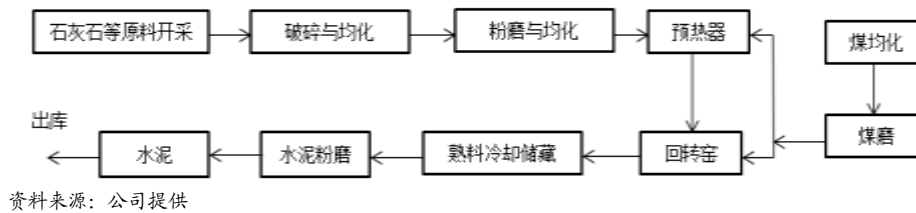
图6 公司水泥生产工艺流程图
