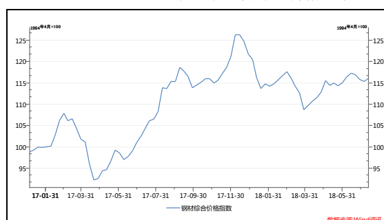
图2 2016年以来钢材综合价格指数
