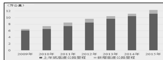
图1 2009~2015年中国高速公路通车里程
