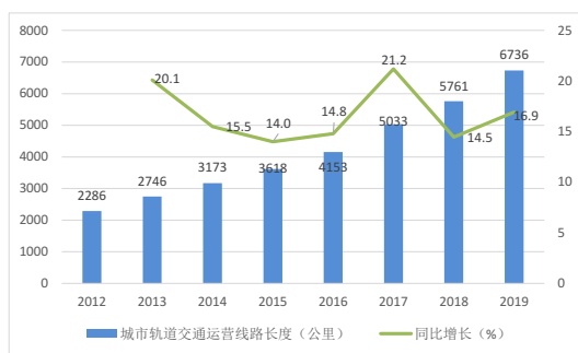
图1 2012-2019年中国城市轨道交通运营里程
