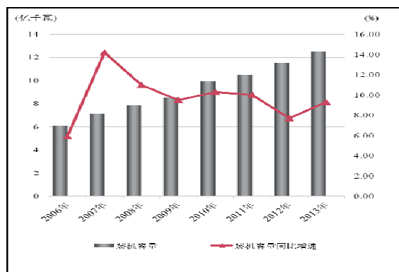
图6 2006~2013年中国发电装机容量变动情况
