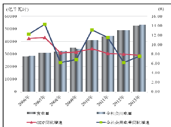
图7 国内发电量、全社会用电量及增幅情况
