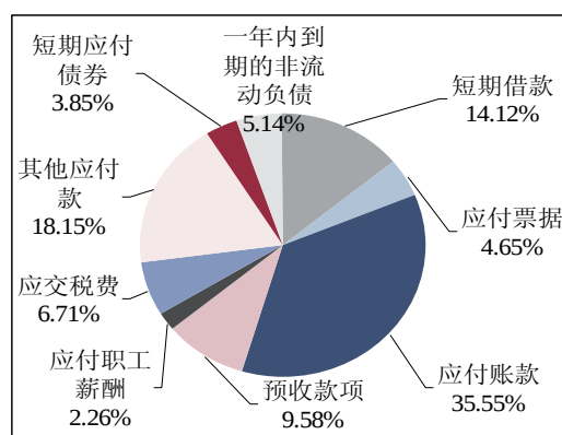
图 5 2007 年底公司流动负债构成
