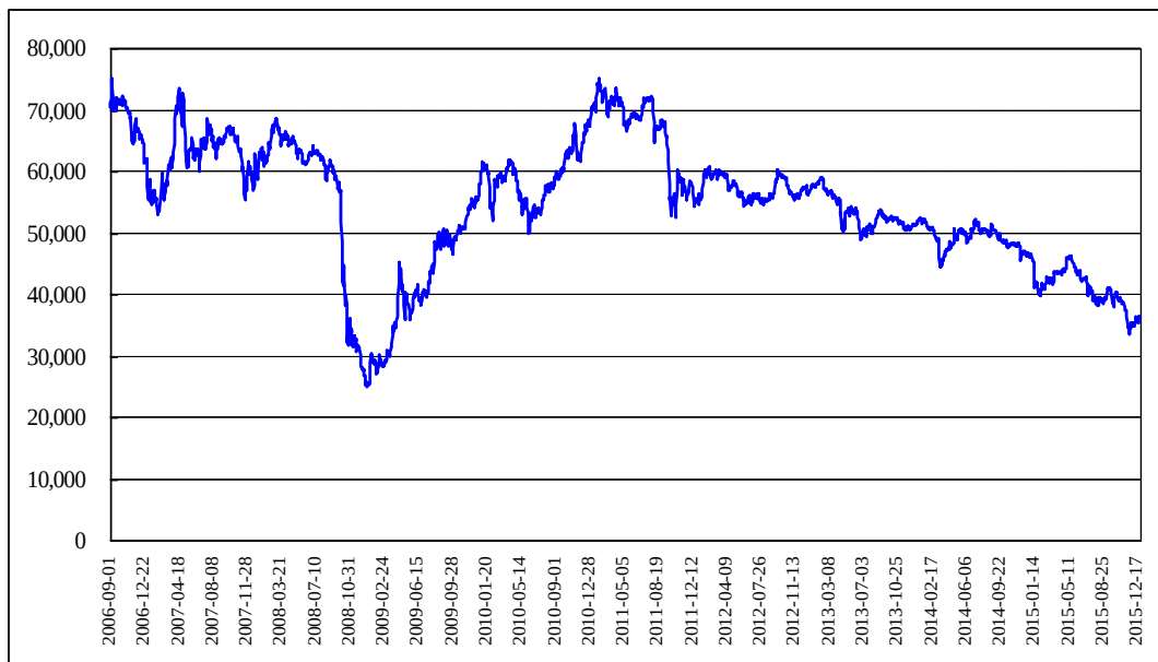
图3 2006年9月~2015年12月年电解铜价格走势（单位：元/吨）
