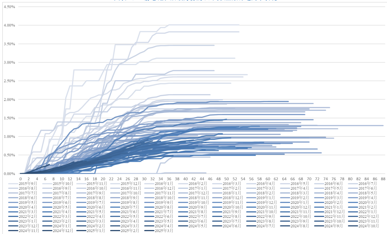
图表 10 · 静态池在后续月份的 30 天以上累计违约率表现
