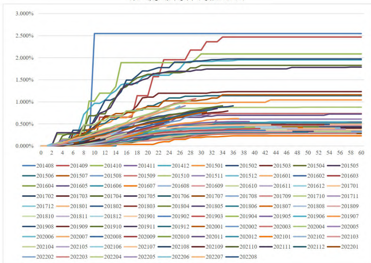
图 2 静态池累计违约率（逾期 30 天以上）
