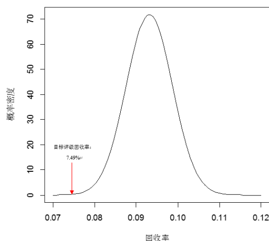
图4 回收概率分布图
