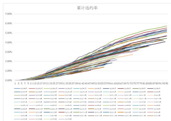
图 4 静态池在后续月份的 90 天以上累计逾期率表现
