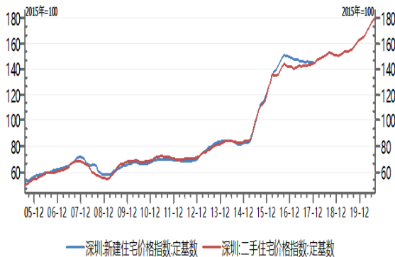
图 3 深圳市新建商品住宅和二手住宅价格指数：定基数
