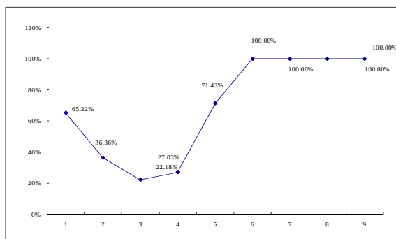
图 3 各期单户最大还本额与还本总额的比例
