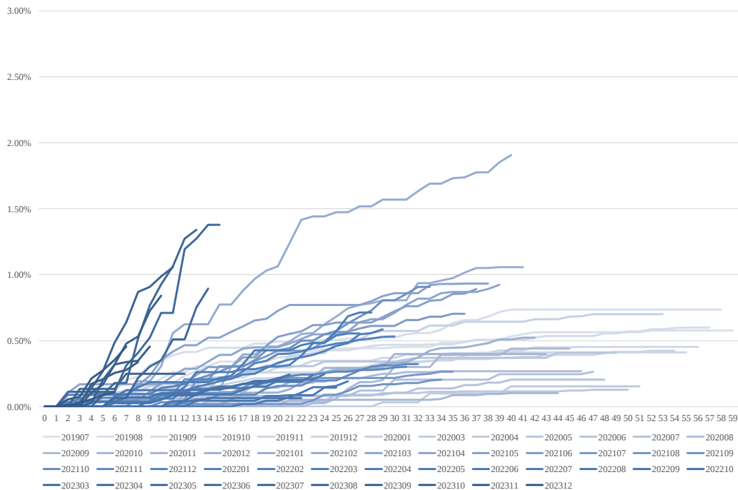
图表 15 • 静态池在后续月份的 30+ 累计违约率表现图
