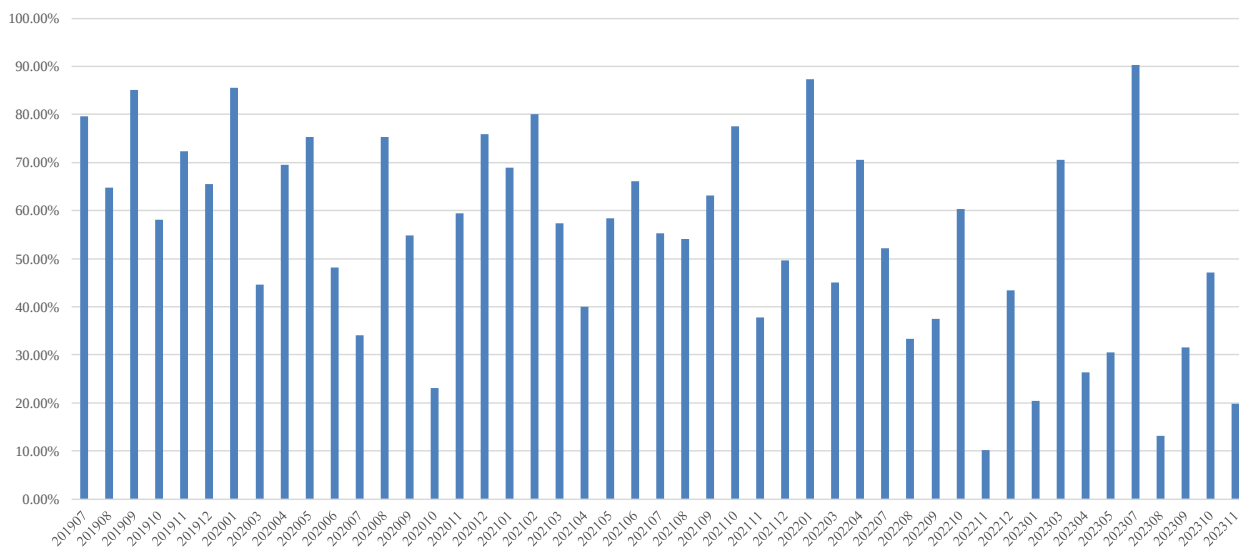
图表 16 • 静态池回收率分布
