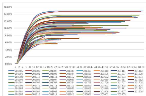
图2 静态池在后续月份的30天以上累计逾期率表现
