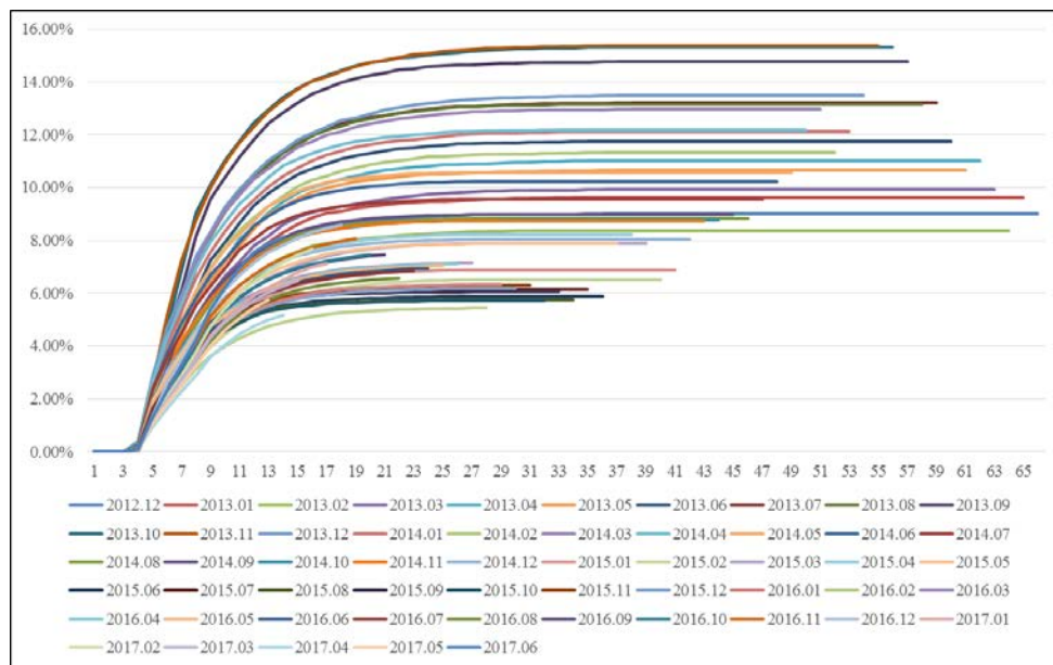
图 2 静态池累计违约率（拖欠 91-120 天）
