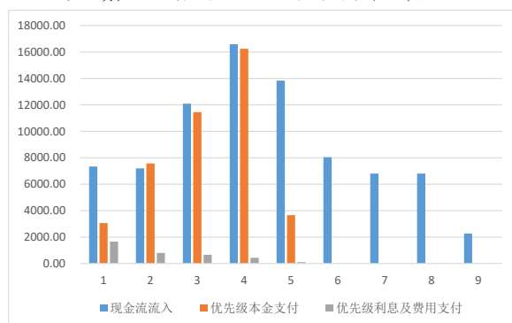
图8 资产池预期回收金额及回收时间分布(单位:万元)
