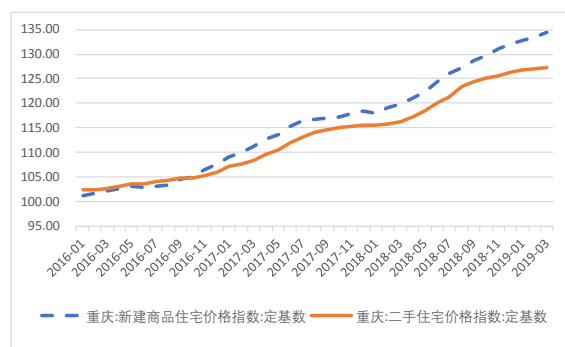
图 2 重庆市新建商品住宅和二手住宅价格指数: 定基数 数据来源: Wind 资讯
