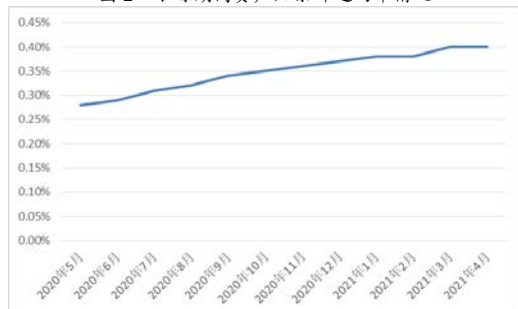
图 2 跟踪期内资产池累计违约率情况
