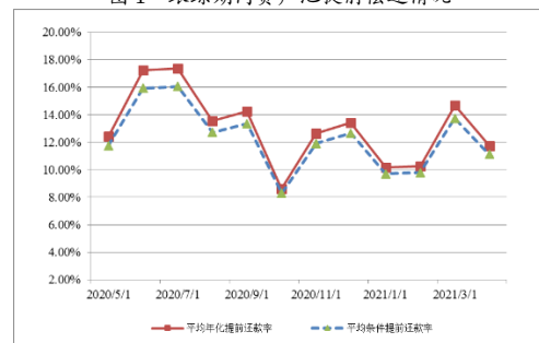
图 1 跟踪期内资产池提前偿还情况
