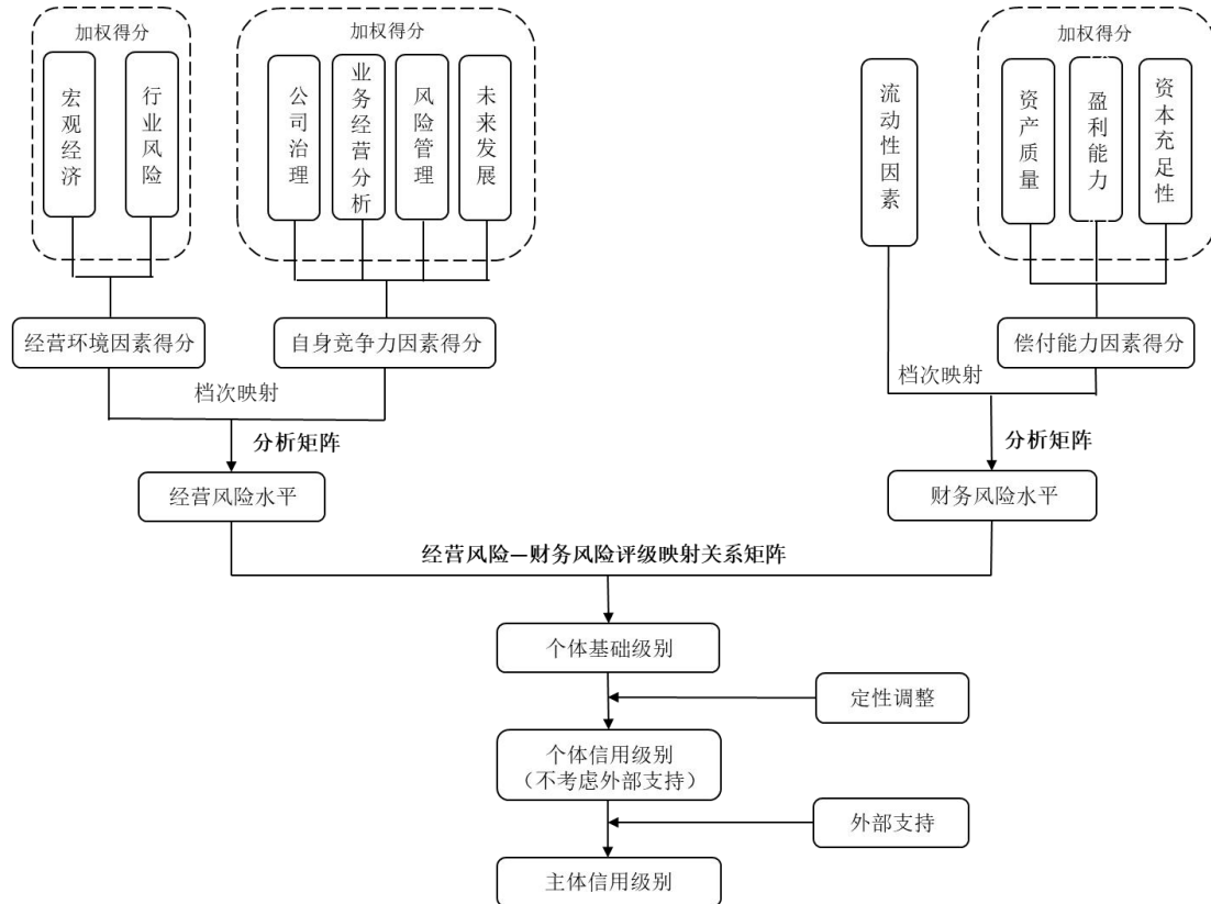
图 1 融资租赁企业主体信用评级打分表架构图
